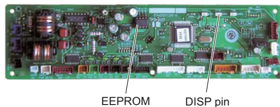
A747336 : 4-Way Cassette 60 x 60 Type
