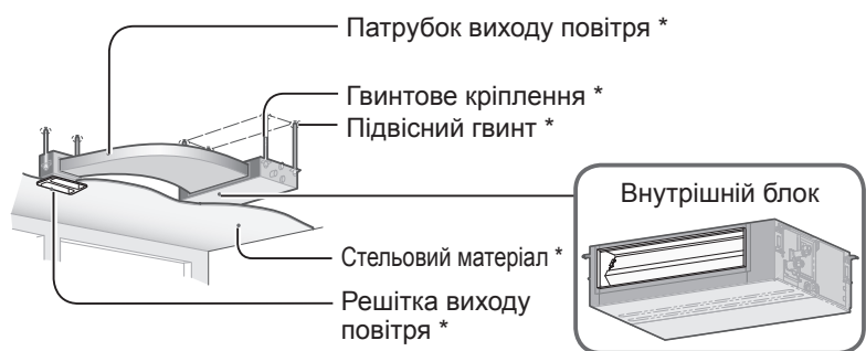
Тип U2 (Низькопрофільна каналізація)
