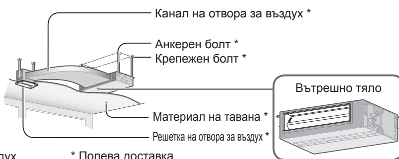
Тип F2 (Компактен с канал)
