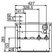
ΚΑΤΩ ΟΨΗ
