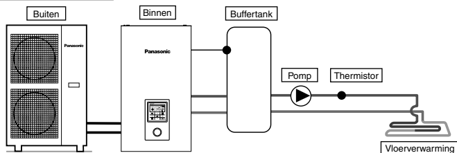
Aansluiting buffertank
