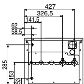
POHLED ZEŠPODA
