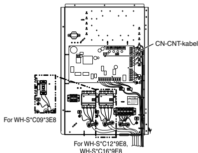
Uten alternativt krets-kort
