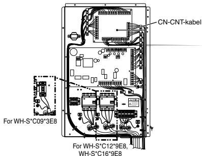
Med alternativt krets-kort
