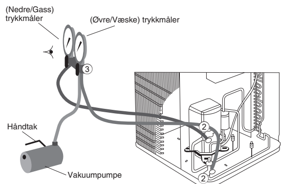
Eksempel på innstilling for deteksjon av kjølemediumlekkasje.
