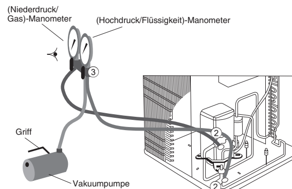
Die Beispiel-Abbildung zeigt ein Setup zur Erkennung von Kältemittel leaks.
