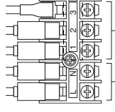
Cavo di alimentazione tra unità interna ed esterna
