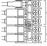
Güç beslemesi (dış ve iç ünite arasındaki bağlantı kablosu)
