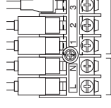
Καλώδιο ηλεκτρικής παροχής μεταξύ εξωτερικής και εσωτερικής μονάδας
