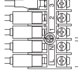
Καλώδιο σύνδεσης ηλεκτρικής παροχής (μεταξύ εξωτερικής και εσωτερικής μονάδας)
