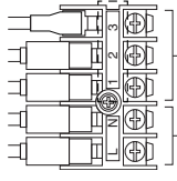
Cavo di collegamento tra unità interna ed esterna
