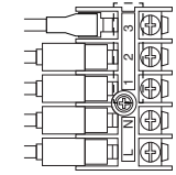
Stromversorgungskabel Verbindungskabel zwischen Außen- und Inneneinheit
