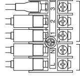
Câble de raccordement entre l'unité intérieure et extérieure
