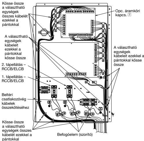
A választható kábelek és a tápkábel vezetésének módja (belső vezetékvezetés nélküli nézet)
