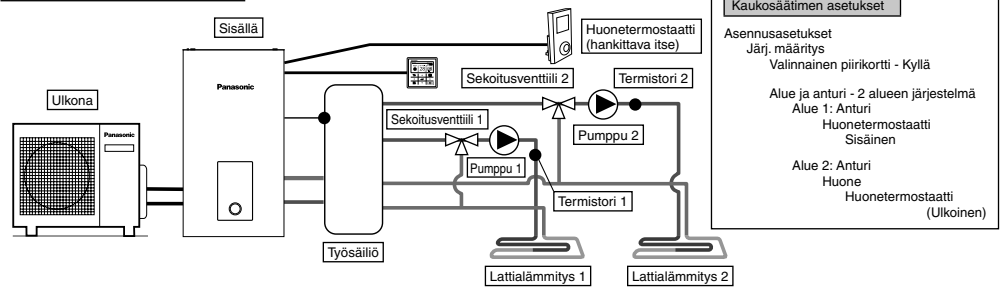
Lattialämmitys 1 + Lattialämmitys 2
