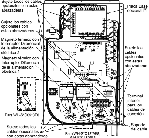
Cómo guiar los cables y el cableado de alimentación de la instalación (vista sin el cableado interno)
