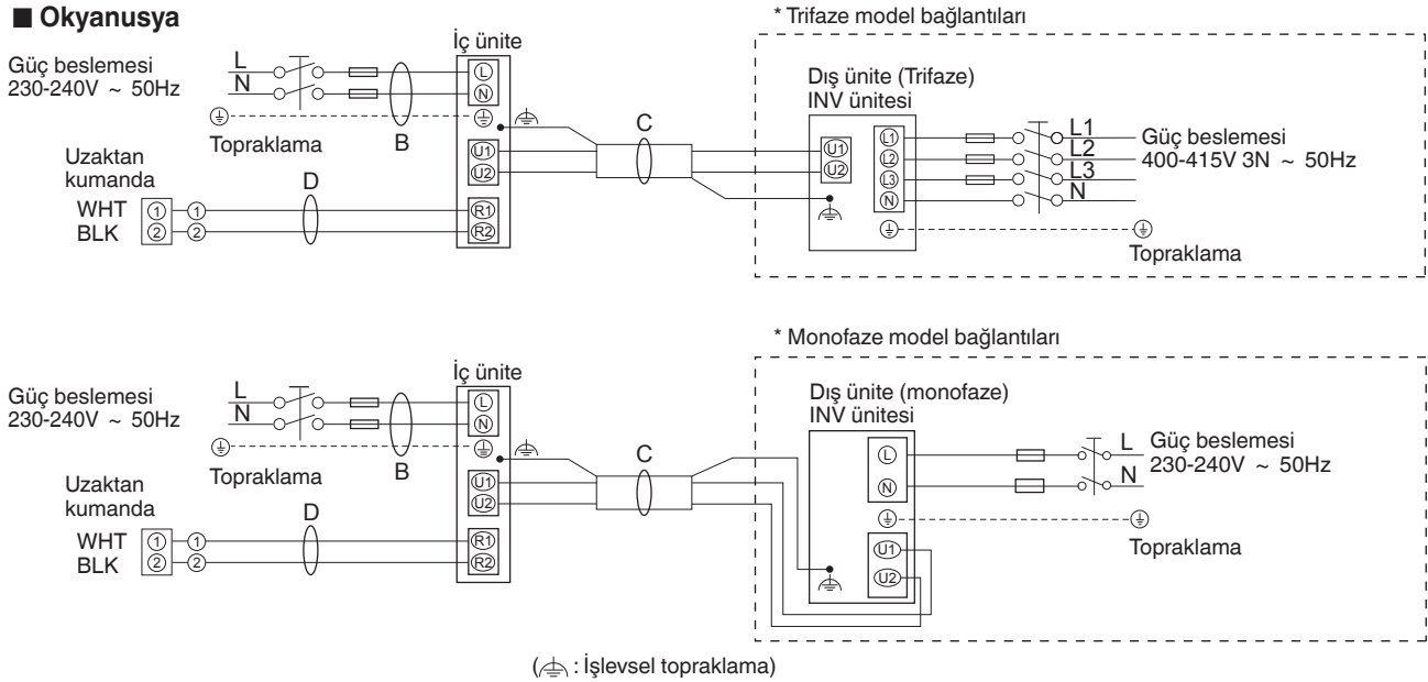
6P terminal kartı
