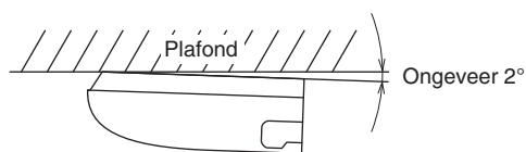
Diagonaal achter (zijaanzicht)
