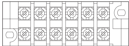
L N U1 U2 R1 R2 Güç beslemesi Üniteler arası kumanda kablosu Uzaktan kumanda kablosu Tip T2
