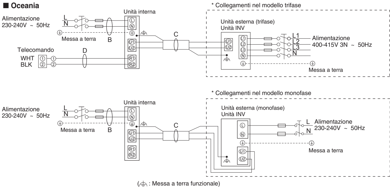
Scheda dei terminali a 7P
