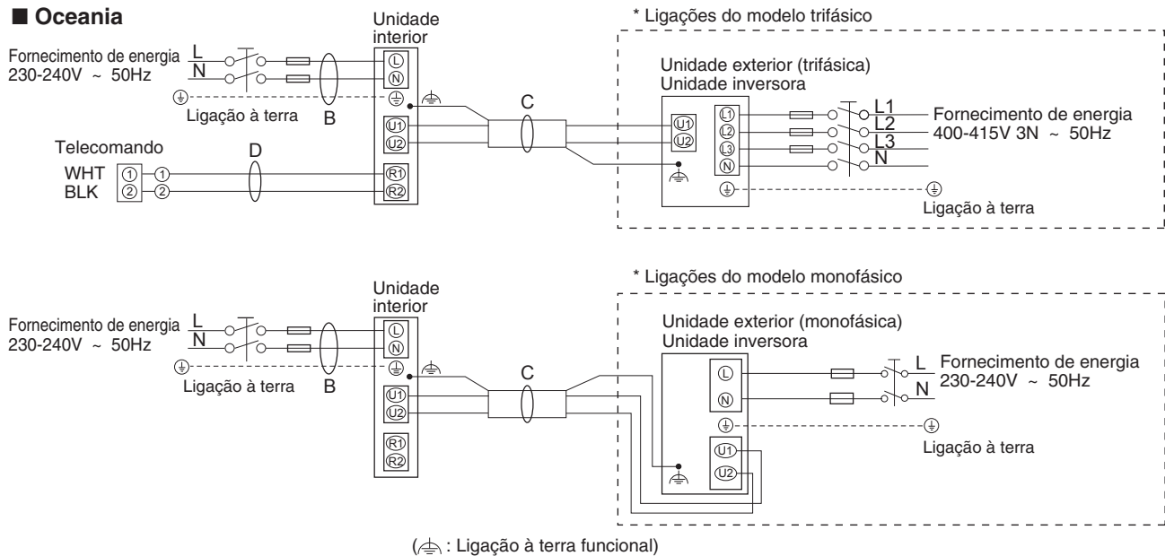
Quadro de terminais 7P
