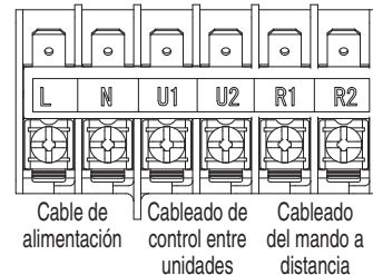
Tarjeta de terminales
