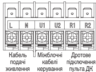
Панель роз'ємів
