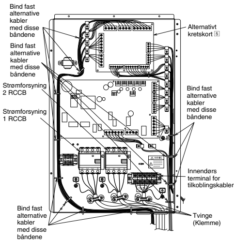
Hvordan trekke de ekstra kablene og strømledningen (vist uten intern kabling)
