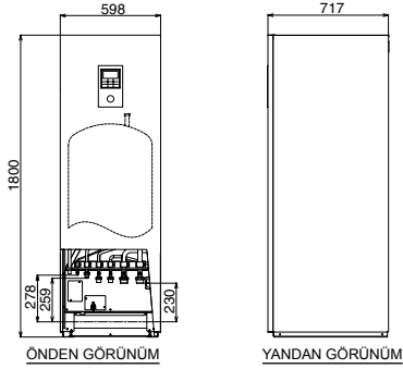
ÖNDEN GÖRÜNÜM
