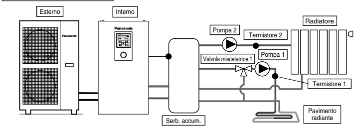
Pavimento radiante + Radiatore
