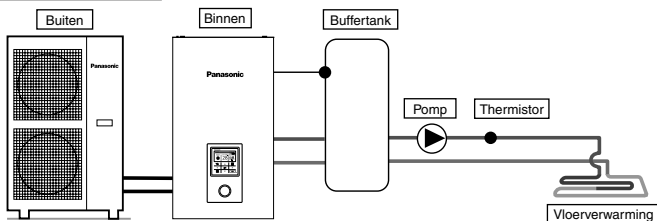
Aansluiting buffertank
