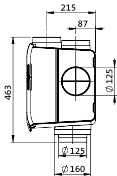
Fig. 2 Zijaanzicht MVS-15
