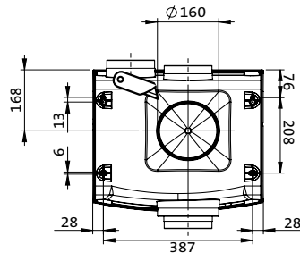
Fig. 5 Achteraanzicht met Ø160mm aansluiting
