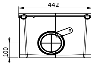
Fig. 6 Onderaanzicht met Ø125mm en Ø160mm aansluiting
