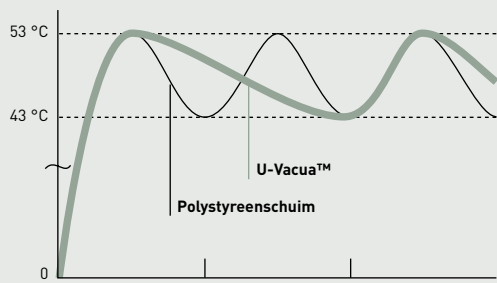
Watertemperatuur tank
